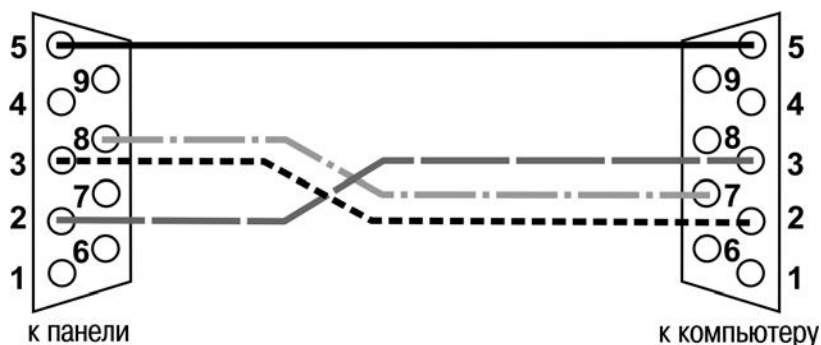
Рис. 5.2. Схема нуль-модемного кабеля для конфигурирования панели ИП320 с переходником
