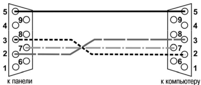
Рис. 5.2. Соединительный кабель для конфигурирования панели ИП320 без переходника
