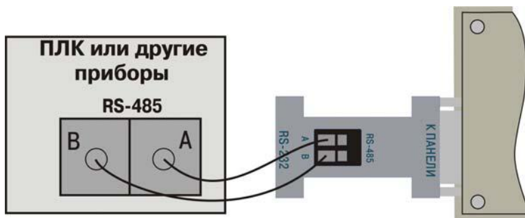
Рис. 6.1. Схема подключения интерфейса RS485 для конфигурирования панели ИП320
